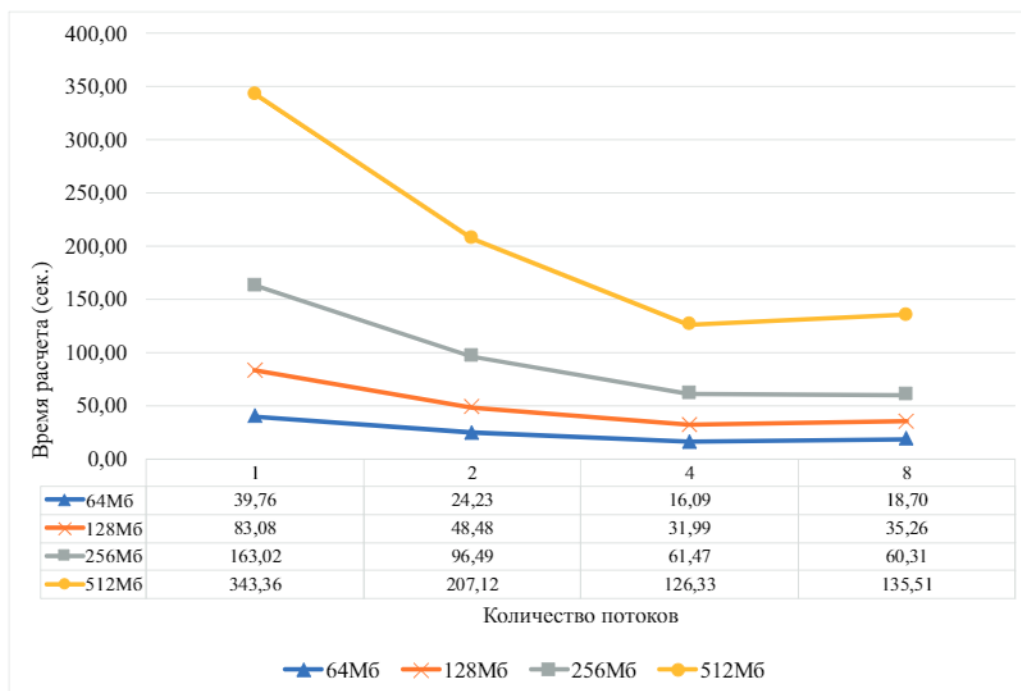
Рисунок 3 – Время вычисления
